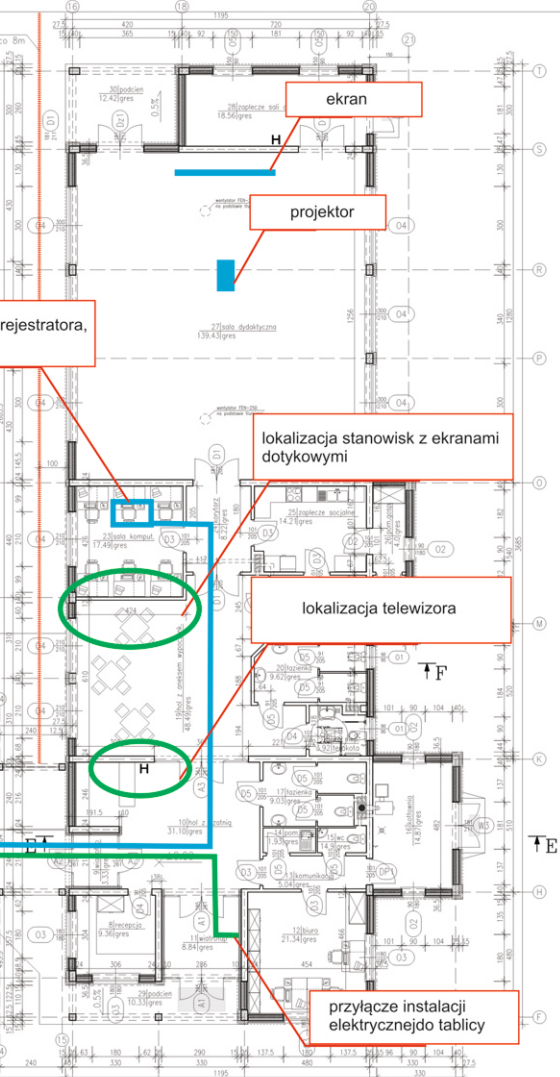
zagroda pokazowa żubrów rzut przyziemia 1:100
