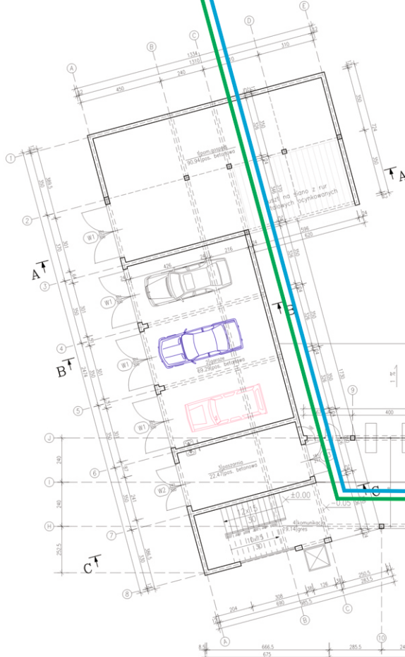
zagroda pokazowa żubrów rzut przyziemia 1:100
